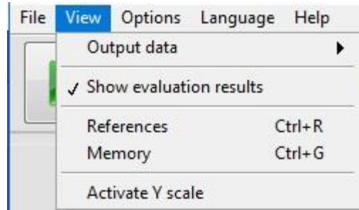
View menu.
